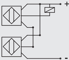
Reihenschaltung
