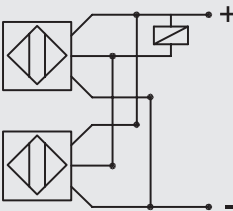
Conexión en paralelo
