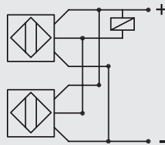
Parallelschaltung
