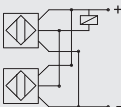
Montage en parallèle
