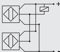
Connessione in parallelo
