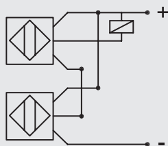
Montage en série
