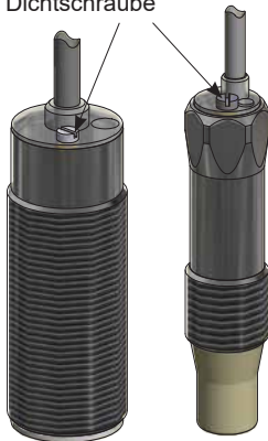
Dichtschaube
