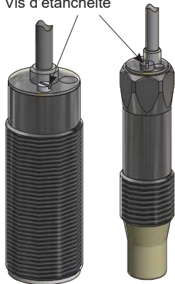
Vis d'étanchéité
