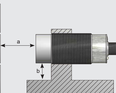
Fig. 4 Non noyable
