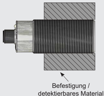
Abb. 1 Bündig montiert
