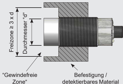
Abb. 2 Nichtbündig montiert
