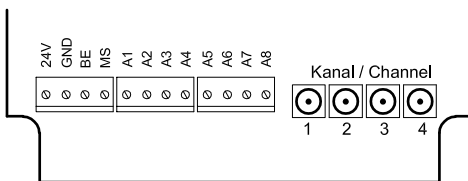
Anschlussbild
