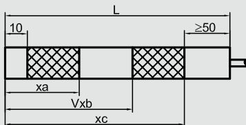
Abb. 3 KFS-4-.../KFX-4-... Sonde mit variablen Grenzwertschaltpunkten
