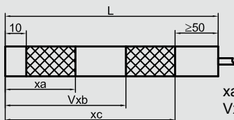
Figura 3 KFS-4-.../KFX-4-... Sonda con puntas de medición variables.
