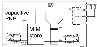
Sonda a 2 punti PNP / MM
