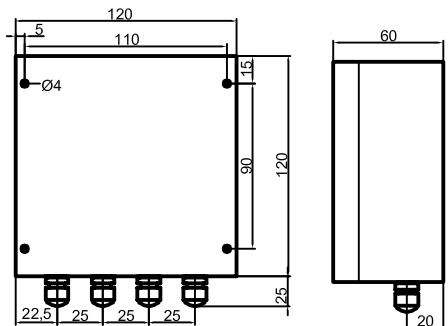
Maßskizze
