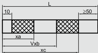
Fig. 3 Sonde KFS-4-.../KFX-4-... avec seuils variables
