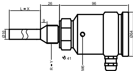
Fig. 3: Tête de connexion en acier inox VA
