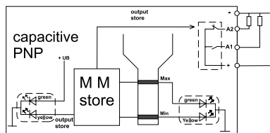
Sonda de 2 puntos PNP / MM
