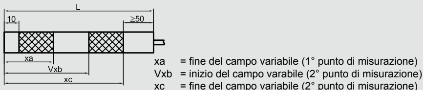
Fig. 3 KFS-4-.../KFX-4-... Sonda con punti di misurazione variabili
