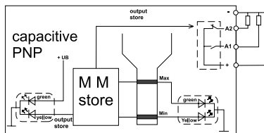
Sonde PNP à 2 seuils / Min.-Max.
