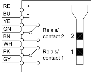
Anschlussbild 3 Relaisausgang
