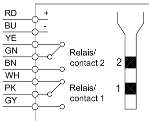
Schéma de raccordement 3 Sortie par relais
