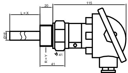
Fig. 4: Tête de connexion en fonte d'aluminium
