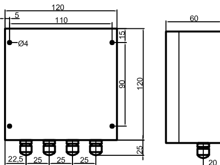
Schéma dimensionnel
