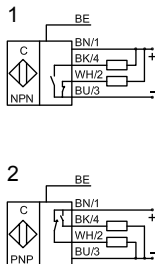
Anschlussbild
