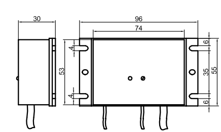
Esquema de dimensiones 2:
