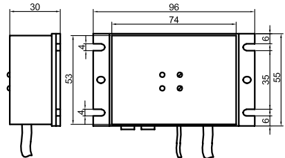
Maßskizze
