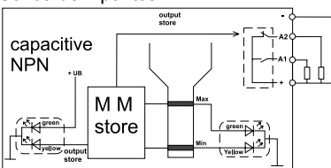
Sonda de 2 puntos NPN / MM
