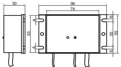
Maßskizze 2
