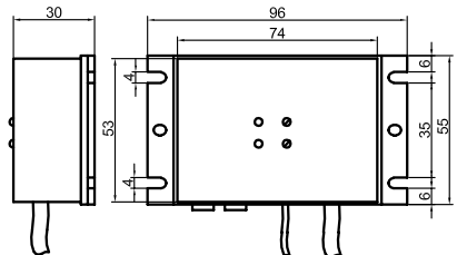
Schéma dimensionnel
