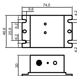
Esquema de dimensiones 1:
