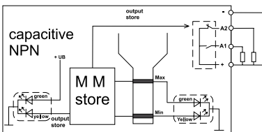
Sonde NPN à 2 seuils / Min.-Max.
