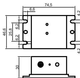
Maßskizze 1
