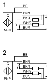
Schéma de raccordement. Fig. 1:
