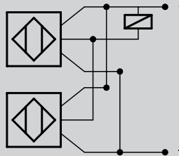
Montage en parallèle
